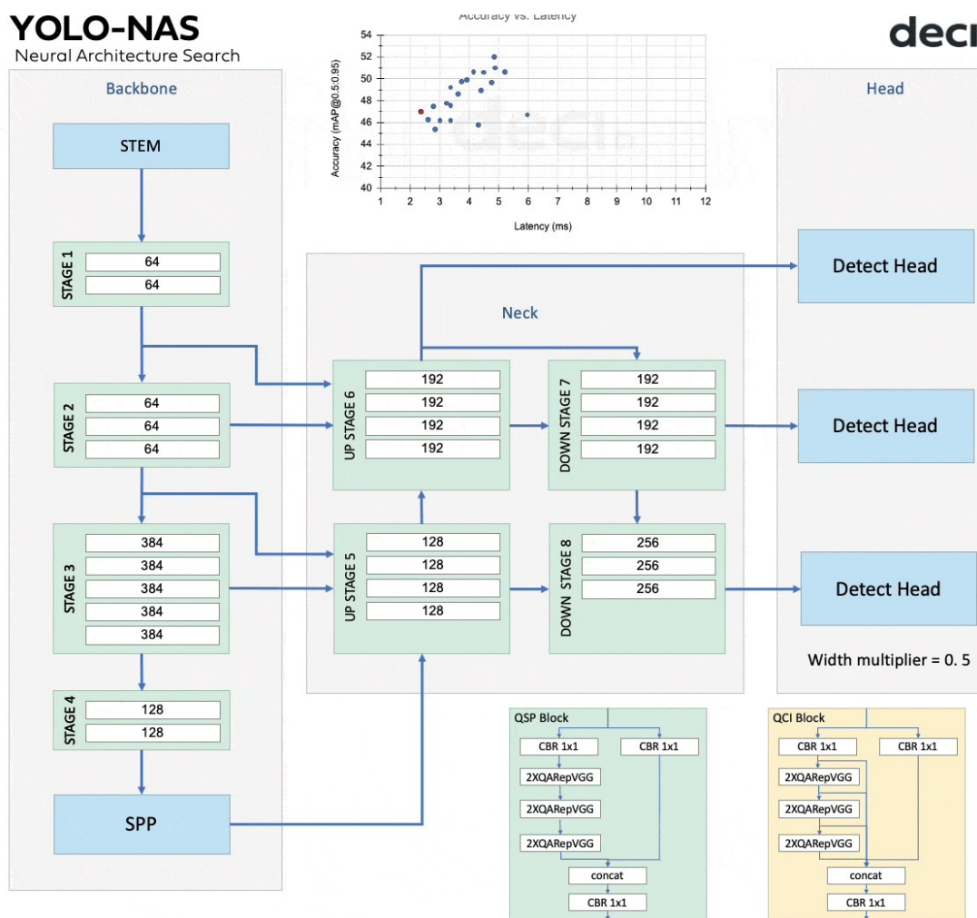
Figura 3.12: Arquitectura YOLO-NAS. La arquitectura óptima se encuentra automáticamente mediante un sistema de búsqueda neural de arquitectura (NAS) llamado AutoNAC para equilibrar latencia y rendimiento.
