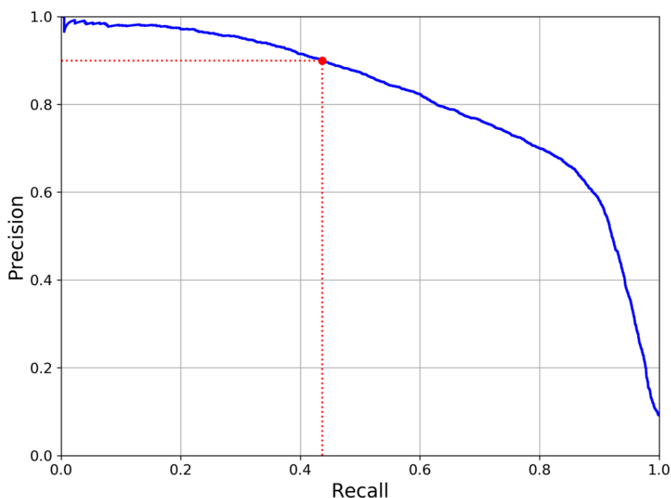
Figura 3.22: Curva de Precision/Recall
